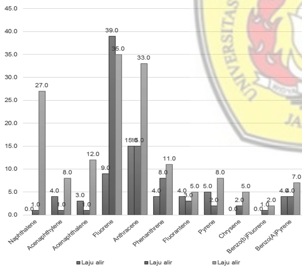
Grafik 1.1 Kandungan PAH pada emisi gas buang kendaraan bermotor pada laju alir gas 30, 45 dan 60 liter per menit selama 50 menit
