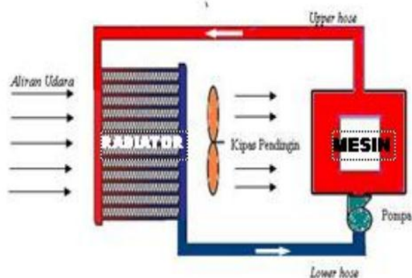
Gambar 2. Skematik radiator
