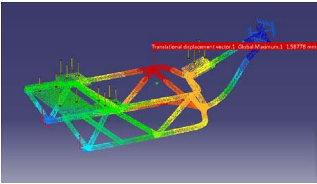
Gambar 13 Vektor displacement pada rangka sepeda
