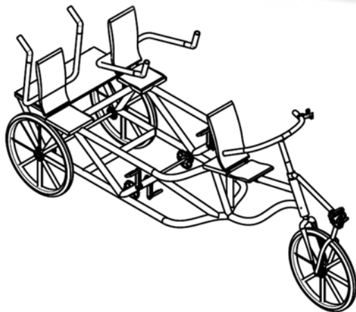
Gambar 14 Desain akhir tampilan isometrik
