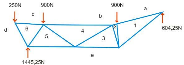
Gambar 9 Freebody diagram 2 Dimensi lengkap dengan gaya eksternal
