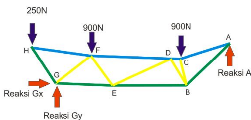
Gambar 7 Penyederhanaan freebody diagram 2 Dimensi
