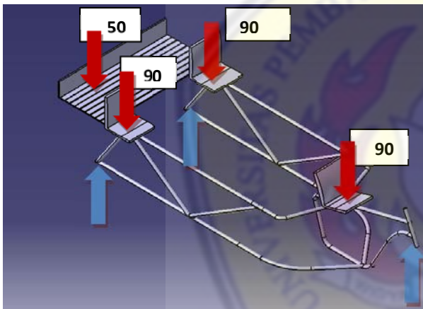
Gambar 6 Peletakan beban aktual
