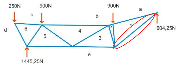
Gambar 11 Bagian kritis ada pada batang 1, ditandai dengan lingkaran.
