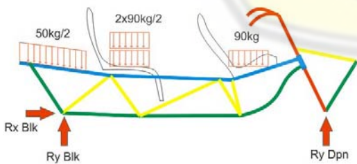
Gambar 7 Penyederhanaan freebody diagram 2 Dimensi
