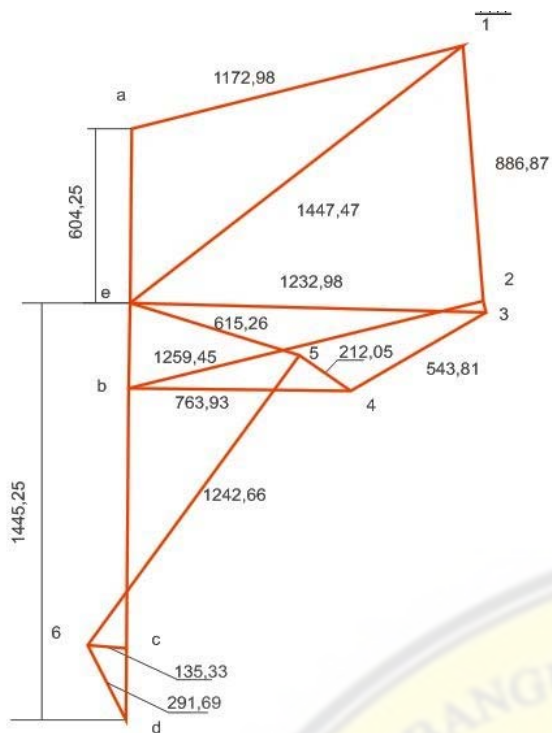
Gambar 10 Grafis vektor gaya pada rangka sepeda
